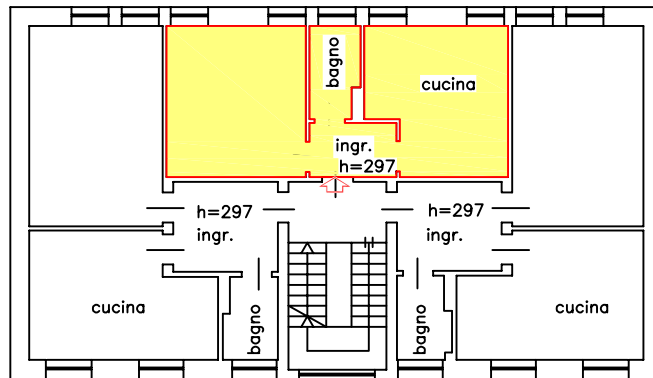
PIANO SECONDO (APPARTAMENTO)
